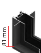
90° Dikey Bağlantı Aparatı Sıvaaltı 90° Vertical Joint Recessed
